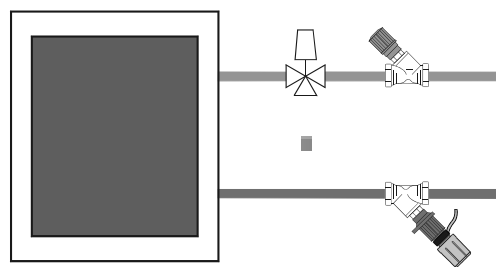
Rys. 7. Kombi-3-plus z silownikiem termicznym w nagrzewnicy / fan coil'u
