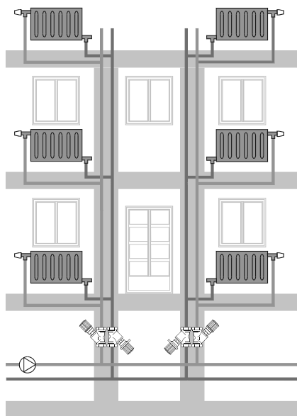
Rys. 4. Kombi-3-plus CZERWONY i NIEBIESKI w pionach
