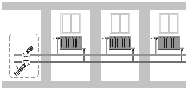
Rys. 5. Regulacja strefowa z Kombi-3-plus z silownikiem termicznym
