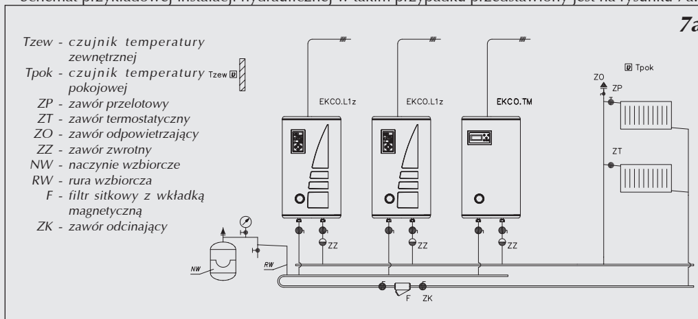
Rys.7a Połączenie grupy kotłów w sieć.
