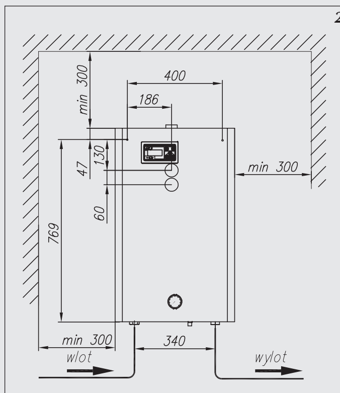
Rys.2 Sposób zamontowania kotła na ścianie.
