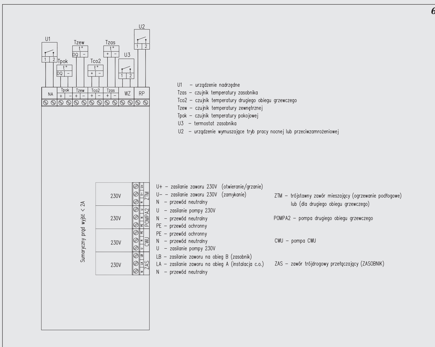
Rys.6 Podłączenie urządzeń zewnętrznych do modułu ZIO
