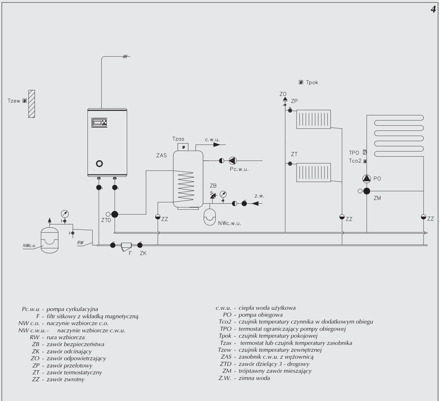
Rys.4 Przykładowa instalacja c.o. z kotłem EKCO.TM – grzejniki, ogrzewanie podłogowe, zasobnik, obieg cwu.
