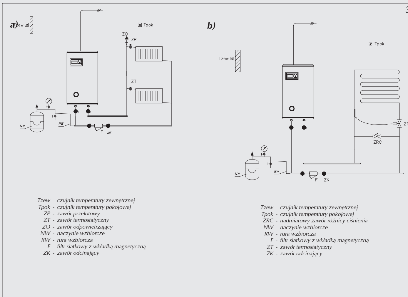
Rys.3 Przykładowa instalacja c.o. z kotłem EKCO.TM
