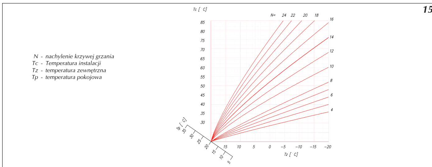
Rys.15 Krzywa grzania.
