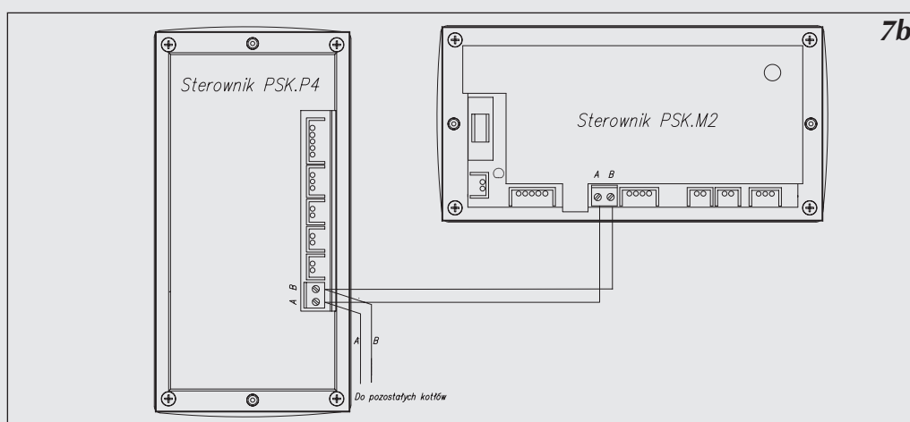
Rys.7b Dodatkowe połączenie elektryczne kotłów pracujących grupowo.
