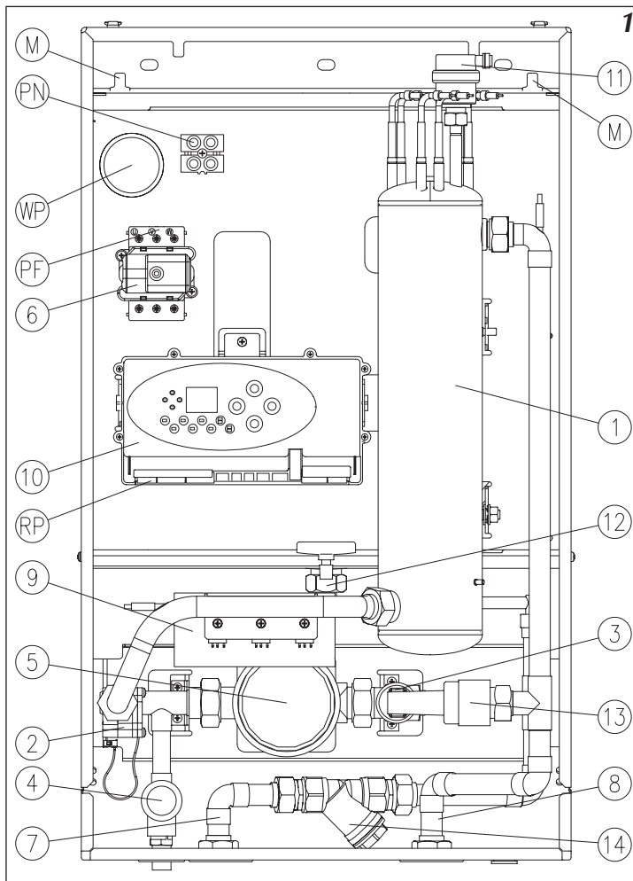
Rys.1 Budowa kotła trójfazowego EKCO.LN2...p
